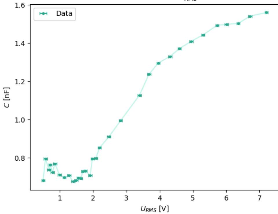
Odvisnost C od U_{RMS}
