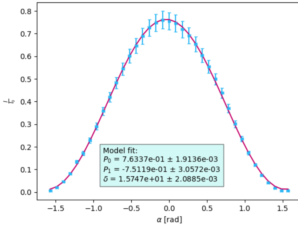
Odvisnost prepuscene moci od kota polarizatorja
