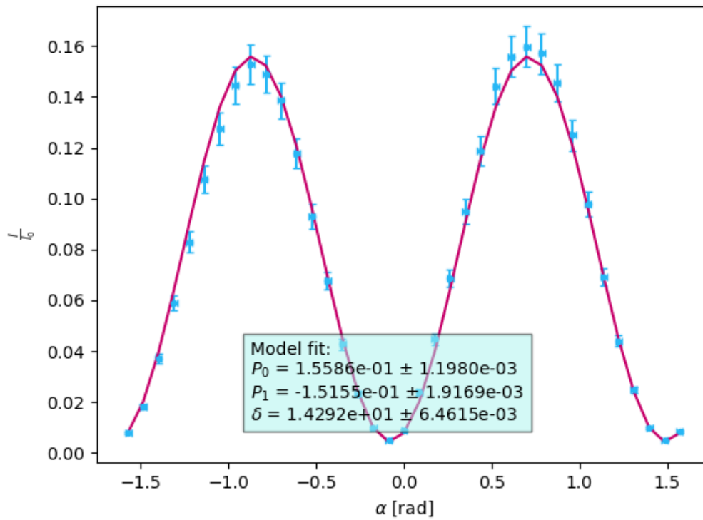
Prepuscena moc v odvisnosti zasuka pol1 glede na pol2
