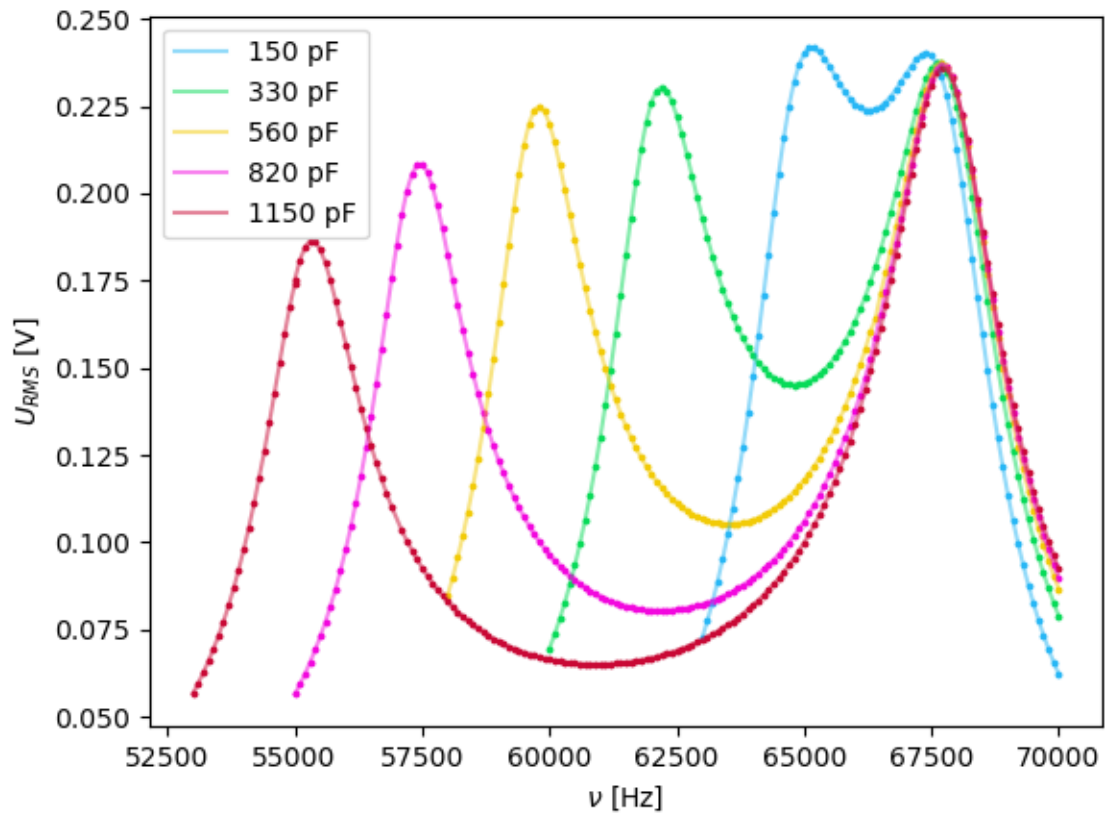
Frekvenca karakteristika
