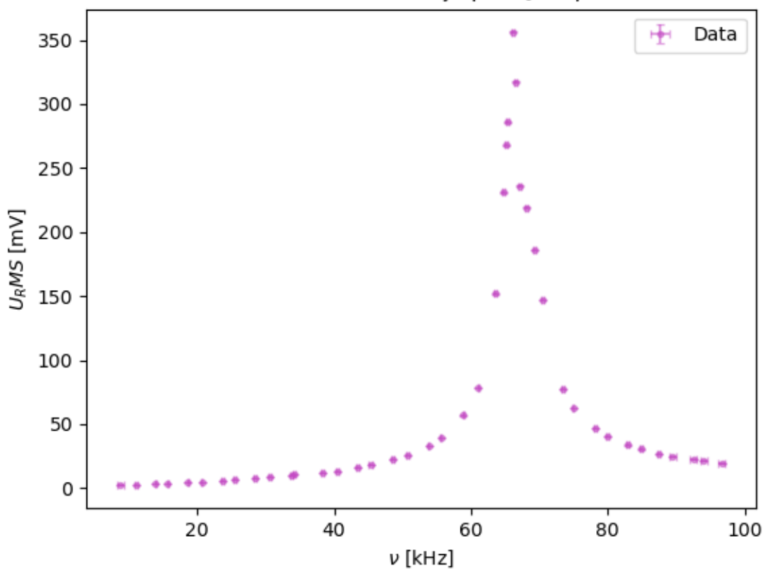
Resonancna krivulja pri C_0 = 0\text{pF}
